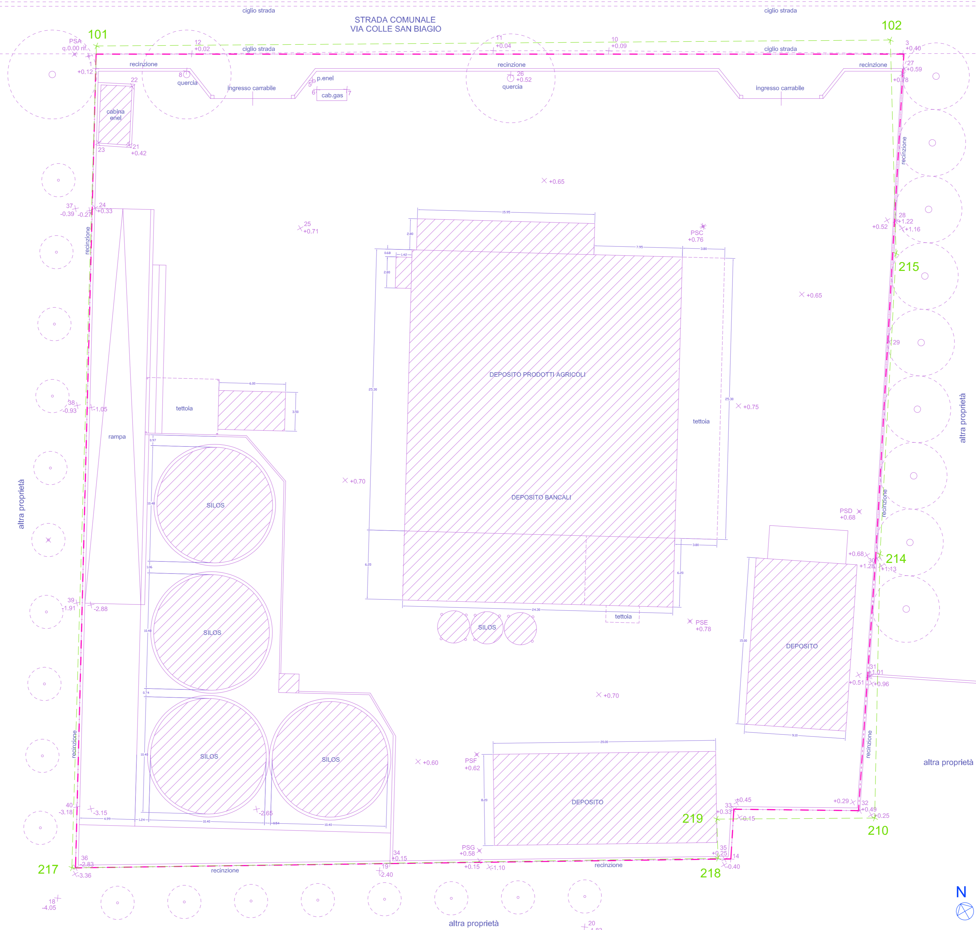
RILIEVO PLANIALTIMETRICO (scala 1:200)
