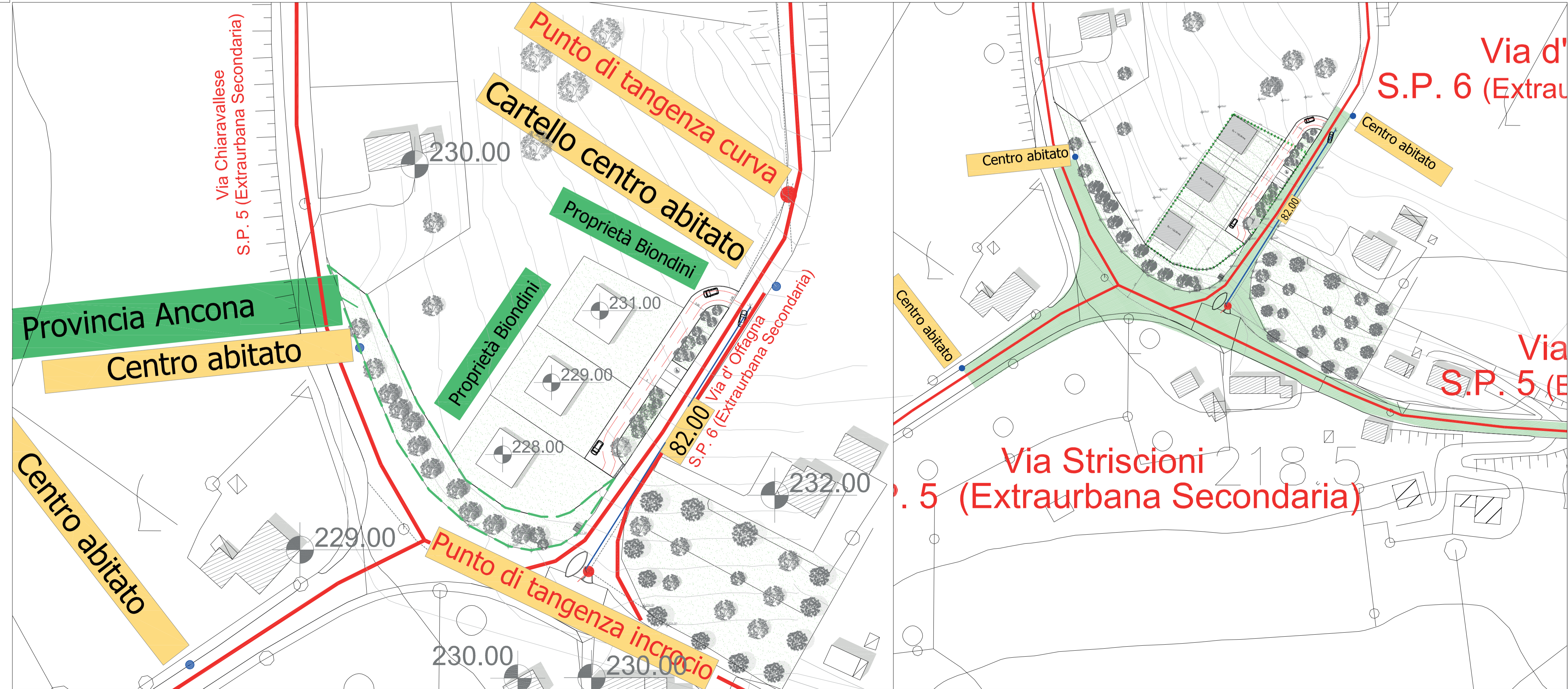
Viabilità e nuovo accesso carrabile Scala: 1:750
