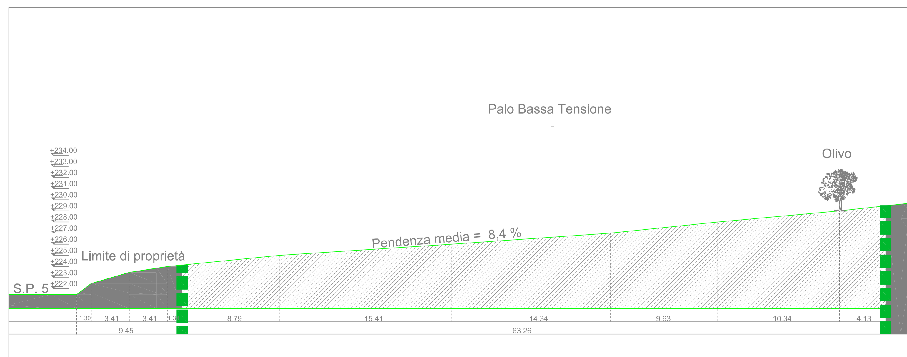
Sez A-A' Scala: 1:200
