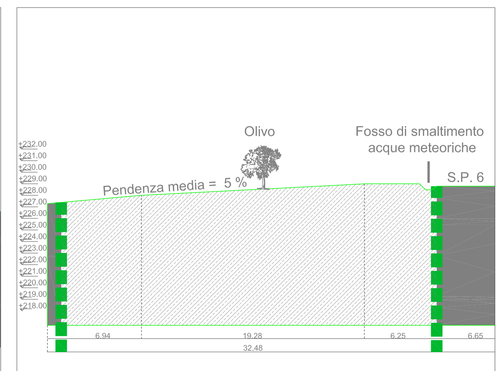
Sez B-B' Scala: 1:200
